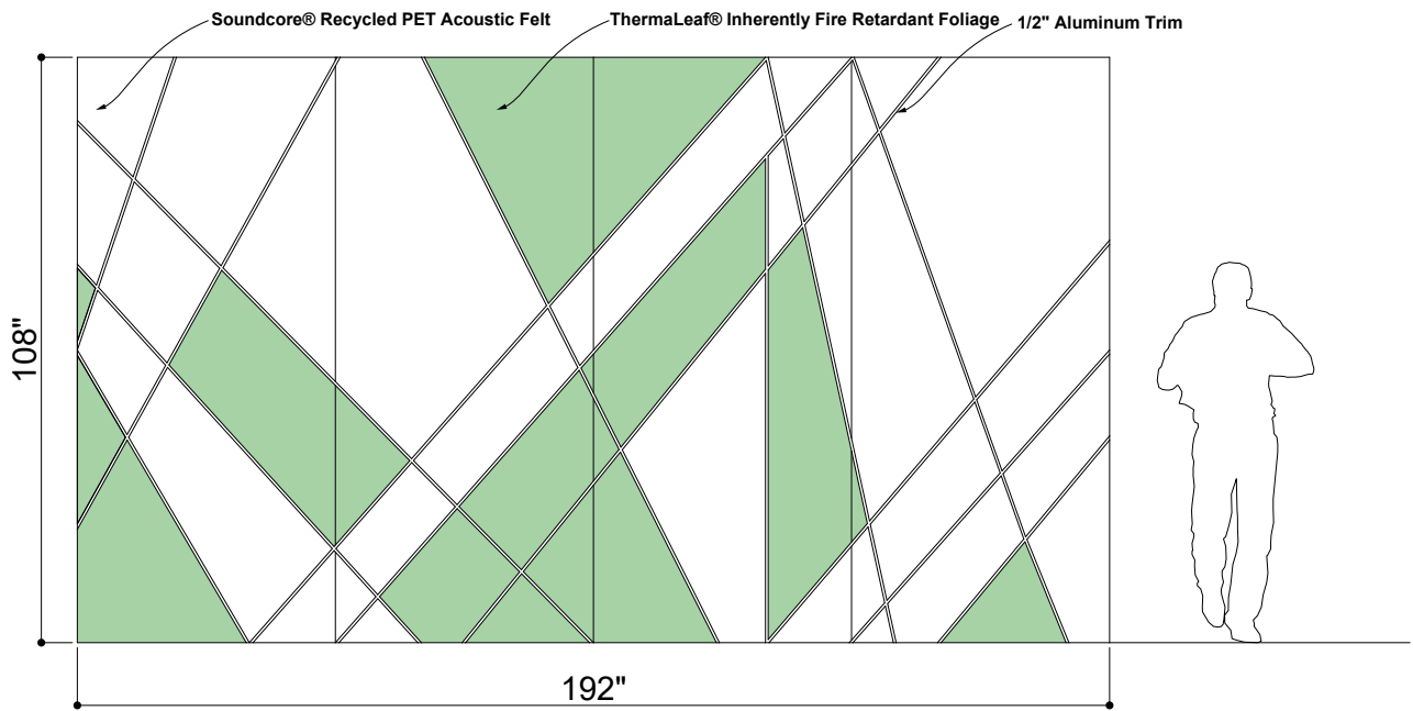
① ELEVATION 2
