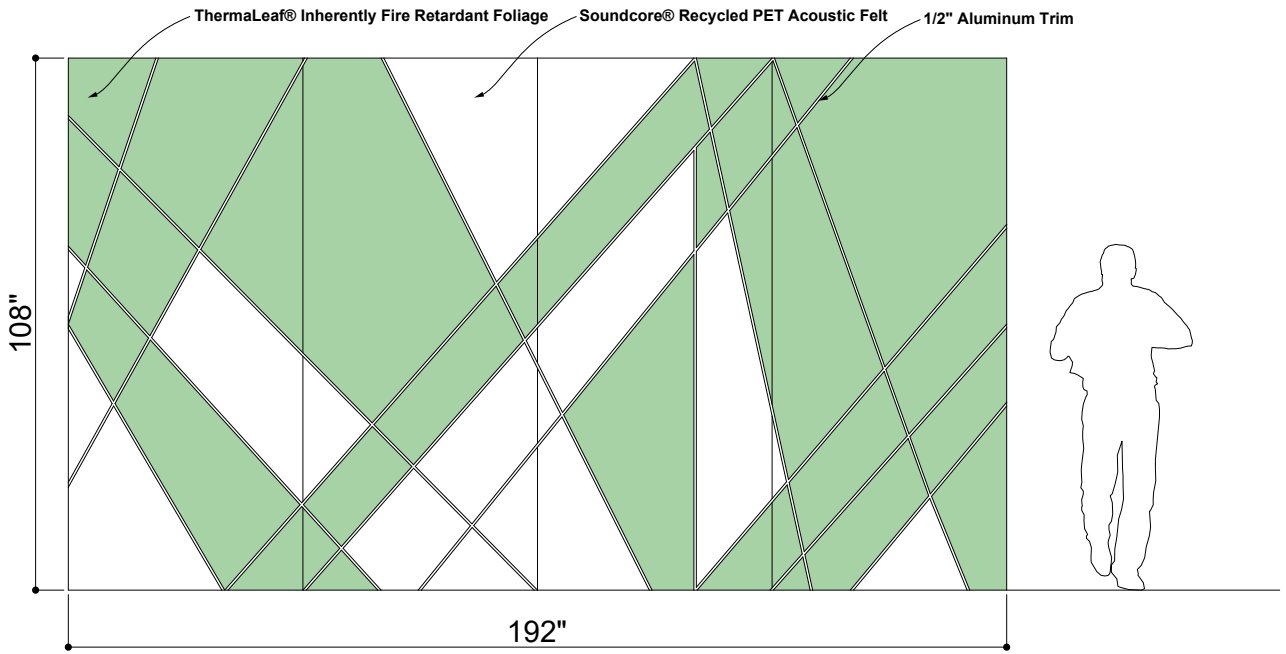
① ELEVATION 1
